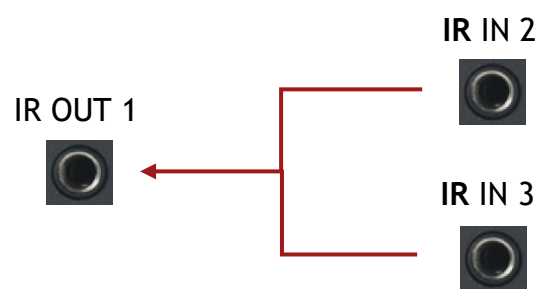
Коммутация ИК-управления
