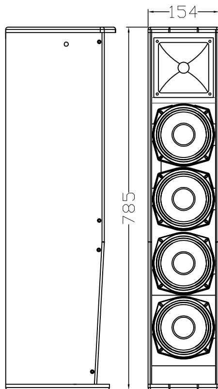
前视图
