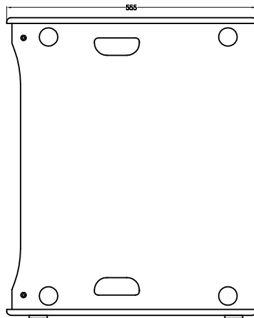
侧视图
