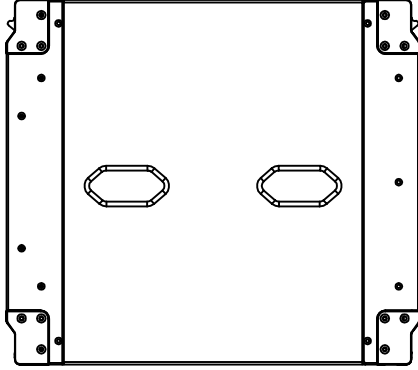
右视图
