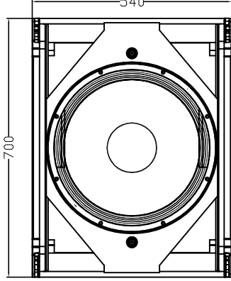
前视图
